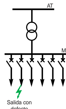
Fig. 3: Eliminación de un defecto monofásico mediante un interruptor automático shunt que al cortocircuitar el defecto permite la extinción del arco.
