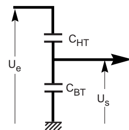
Fig. 37: Esquema de transferencia capacitativa de sobretensiones en el interior de un transformador MT/BT.
