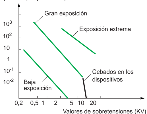
Fig. 11: Número y valor de las sobretensiones estadísticamente posibles según la probabilidad de exposición al rayo.
