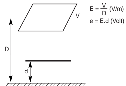
Fig. 32: Ejemplo de campo eléctrico.
