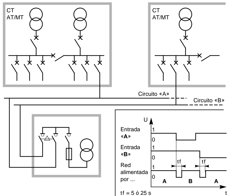
Fig. 5: Alimentación MT de doble derivación. En el cuadro inferior derecho, secuencia del automatismo de un conmutador Merlin Gerin conforme a las especificaciones EDF (Francia).
