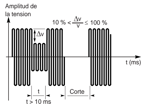
Fig. 1: Bajada de tensión ( \Delta v ) y corte de tensión.
