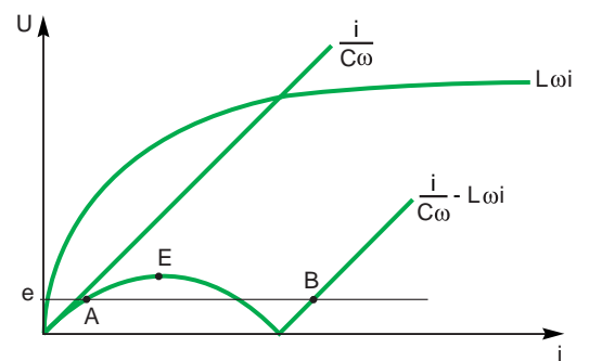
Fig. 39: Principio teórico de la ferorrresonancia.
