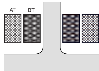
Fig. 36: Posición de los arrollamientos en la columna de un transformador MT/BT.
