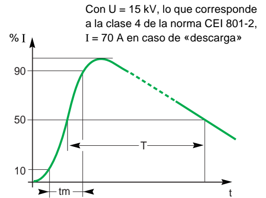
Fig. 35: Corriente de descarga electrostática ( t_m = 5 \text{ ns} ; T = 30 \text{ ms} ).
